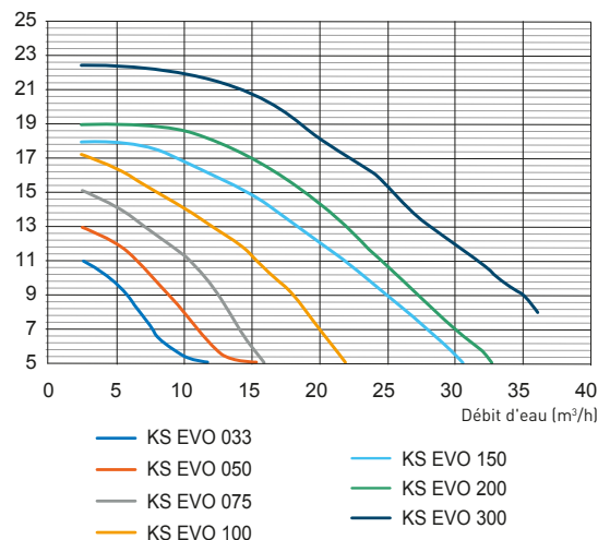
Colonne d'eau (m.) KS Evo / KSX Pro Q (m 3 /h)-H (m)
